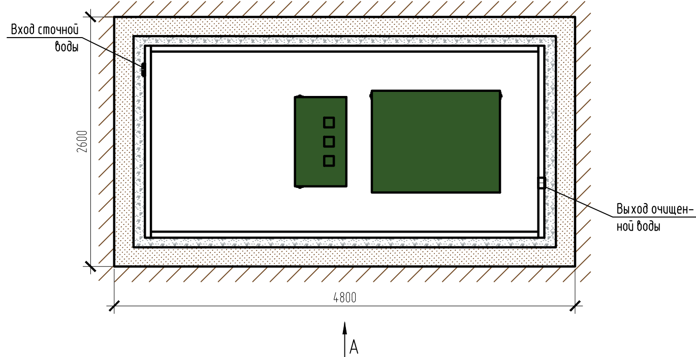
Вид сверху
